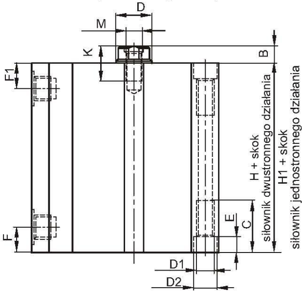
Siłownik z jednostronnym tłoczyskiem
