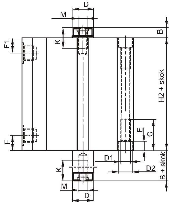
Siłownik z dwustronnym tłoczyskiem
